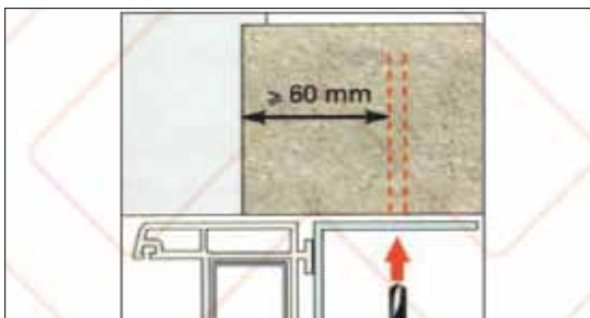
شکل ۵۷ فاصله حداقل پیچ اتصال از گوشه جدار بتنی یا بنایی توپر
