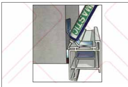
شکل ۶۷ درزبندی پروفیل کناری و فوقانی از طرف داخل
