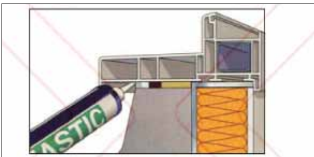
شکل ۶۱ درزبندی زیر پنجره از طرف داخل
