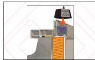
شکل ۵۲ لزوم طراحی و اجرای برای تحمل بار حداقل موضعی (نقطه ای) ۱۰۰کیلوگرمی
