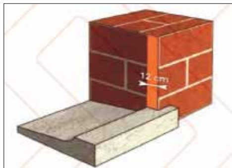
شکل ۴۰ آماده‌سازی سطوح یک درگاه ساخته شده از بلوک یا آجر سوراخ‌دار با تکیه‌گاه پیش ساخته در حالت نصب توکار
