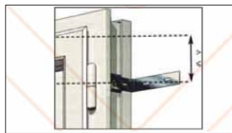
شکل ۴۹ رعایت حداقل فاصله بین نشی‌های اتصال پنجره به دیوار
