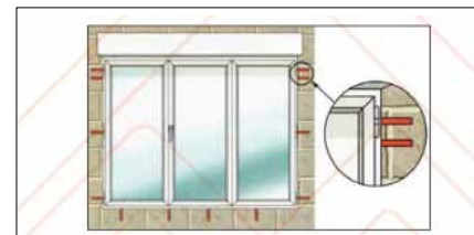
شکل ۵۴ استفاده از نبشی‌های اتصال مضاعف
