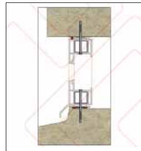
شکل ۷۵ نصب غیر مستقیم پنجره به دیوار توپر بنایی یا بتنی توسط بست و رول پلاگ
