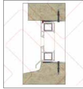
شکل ۷۴ نصب مستقیم پنجره به دیوار توپر بنایی یا بتنی توسط رول بت
