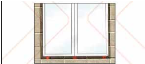
شکل ۴۷ جانمایی لاتن‌های بستر چارچوب
