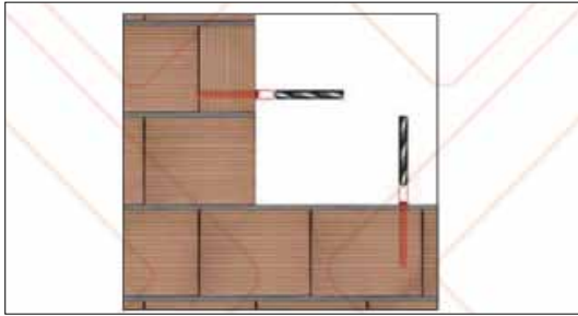
شکل ۷۶ جزئیات اجرایی آماده‌سازی اتصال در صورت اجرای بلوک‌های کناری با حفره‌های قائم
