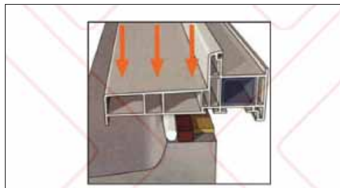
شکل ۶۵ اجرای درزبند خمیری پس از نصب ته‌بند
